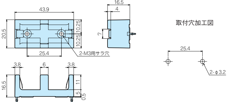
CR123A-R外観寸法図
