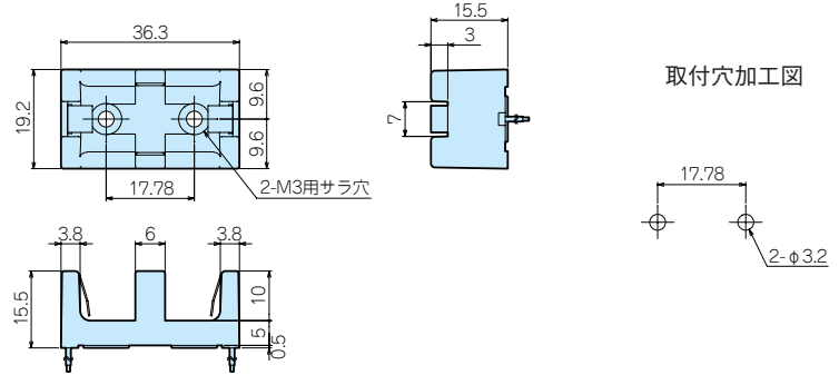
CR2-R外観寸法図
